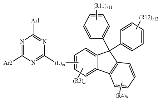
[Formula 3]
